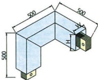
右向异形弯-YR
