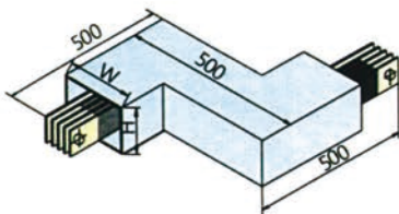
Z形水平弯-ZS
