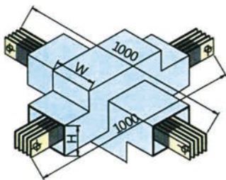
十字形水平弯-SS
