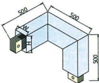
左向异形弯-YL
