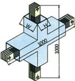
十字形垂直弯-SC
