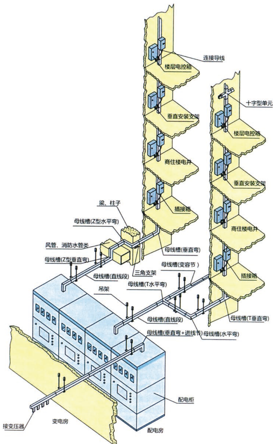
高层建筑总装示意图 Building Assembly diagram
